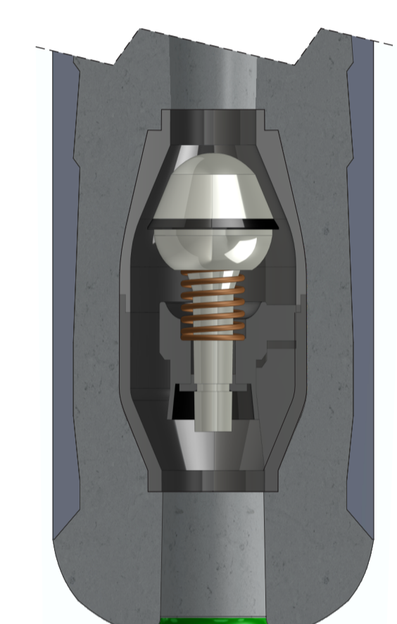
AUTO FILL UP VALVE
