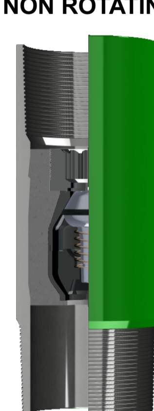
FLOAT COLLAR NON ROTATING
